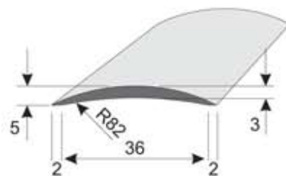
Perfil especial 40 x 5 mm Longitud 6,5 m
