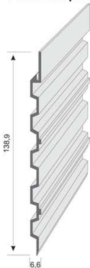
P 9256 Perfil cobertor 139 x 6,6 Longitud 6 m
