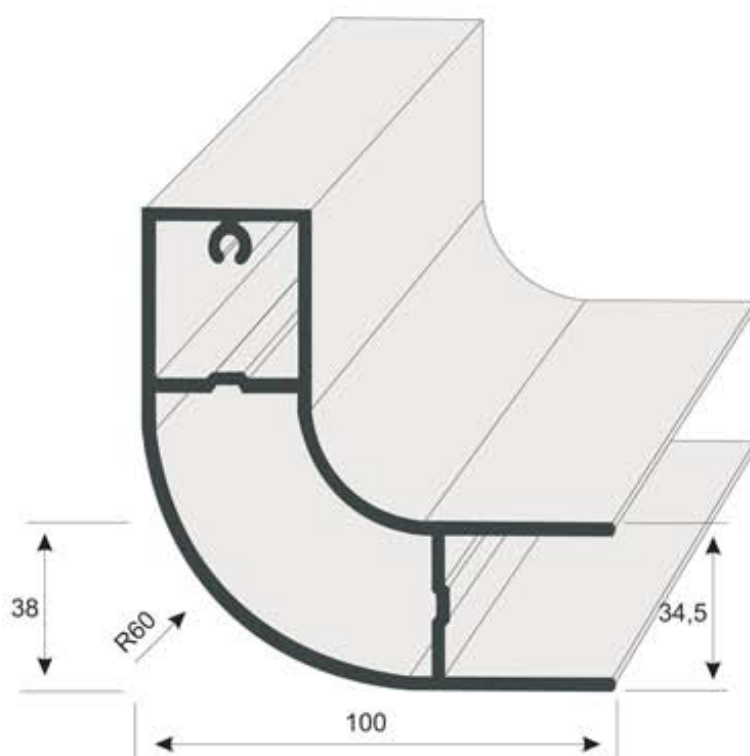
P9160 Perfil cantonero quita miedo 100x100x34,5x1,8 mm Longitud 6 m, anodizado A6C0
