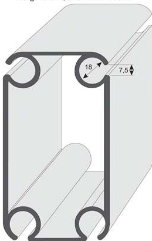
P1374 Perfil para la construcción de carpas 4 listones EN AW 6005A T6, EN 12020-2 130x70x3 mm L= 8 m
