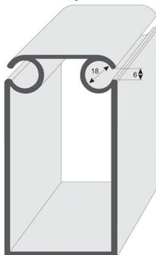
P1372 Perfil para la construcción de carpas 2 listones EN AW 6005A T6, EN 12020-2 130x70x3 mm L= 8 m
