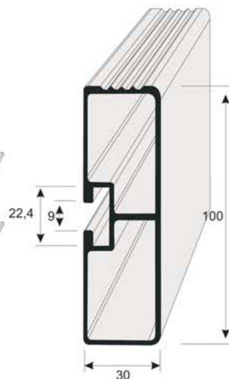
P9161 Perfil quita miedo 100x30x2 mm, anodizado A6C0 Longitud 7,2 m
