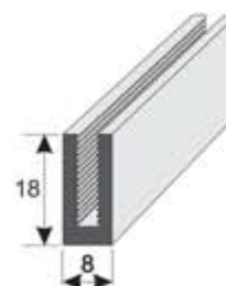
P32 Perfil U para cercados 18x8x2,4 mm Öffnung 3,2 mm
