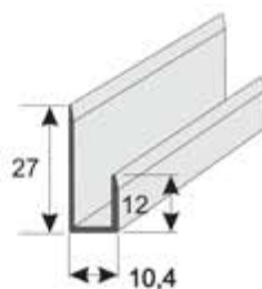
Canal U desigual 27x10,4x12x1/1,2 mm Longitud 6 m
