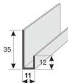
Canal U desigual 35x11x12x1,5 mm Longitud 6 m
