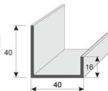
Canal U desigual 40x40x16x2 mm Longitud 6 m
