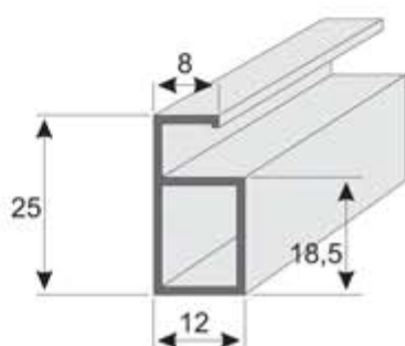
P17 Perfil 6 Longitud 6 m
