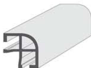
P126 Perfil cantonero 20 x 13 anodizado A6C0 Longitud 6 m
