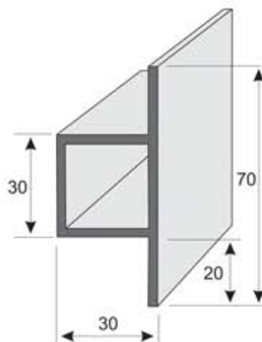
P73 Perfil "Sombrero" 70 x 30 x 30 x 2 Longitud 6 m
