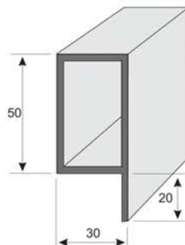
P70 Perfil q 70 x 50 x 30 x 2 Longitud 6 m
