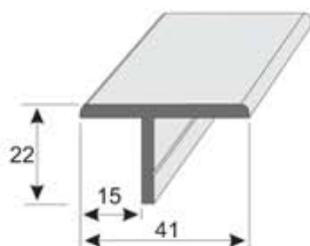
P41 Perfil T 41 x 22 x 3 Longitud 6 m
