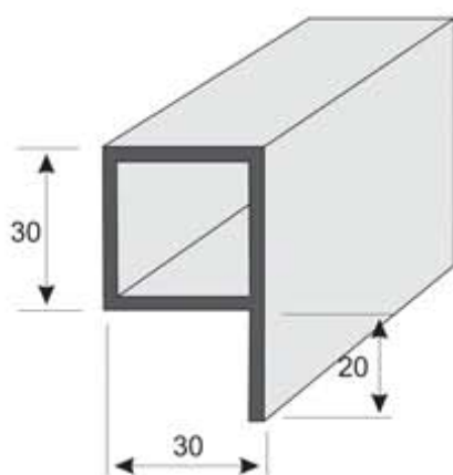
P51 Perfil q 50 x 30 x 30 x 2 Longitud 6 m
