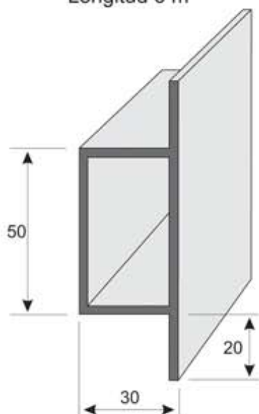
P93 Perfil "Sombrero" 90 x 50 x 30 x 2 Longitud 6 m
