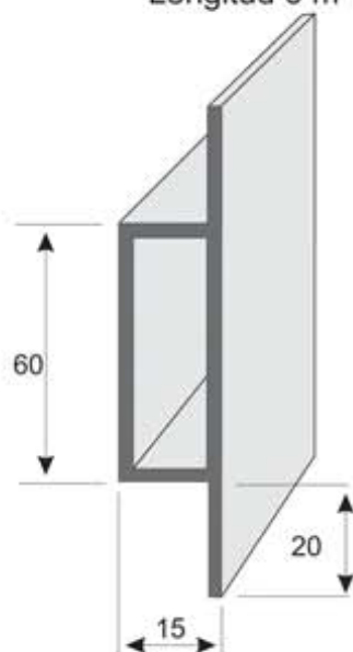
P60 Perfil "Sombrero" 100 x 60 x 15 x 2 Longitud 6 m
