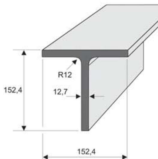
Perfil T 152,4 x 152,4 x 12,7 con radio 12 EN AW 6082 T6, EN 755-9 Longitud 6 m
