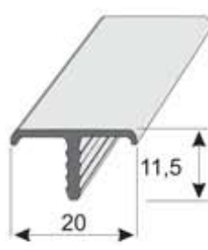
P200 Protector de esquinas anodizado A6C0 Longitud 5 m
