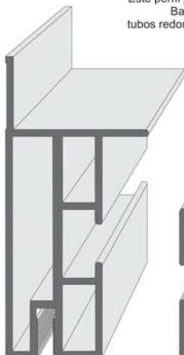
Ha02 Perfil especial 90,20 x 43,50 mm Longitud=6100 mm
