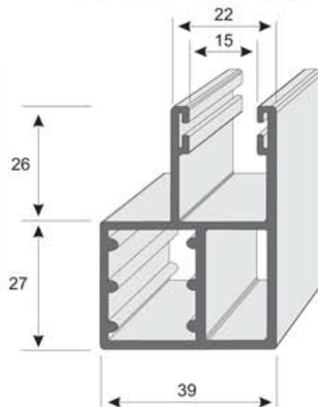
B07 Perfil especial 53 x 39 Longitud 6 m
