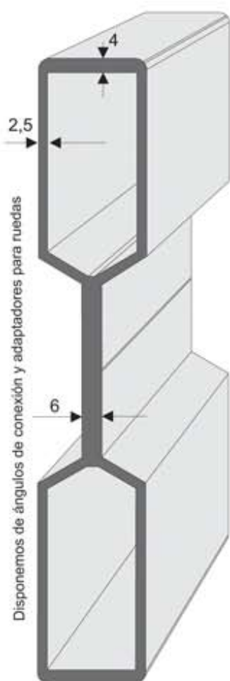
P Z175 Perfil especial 175x30
