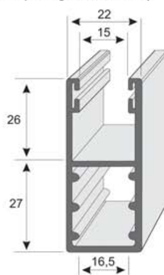
B01 Perfil especial 53 x 22 Longitud 6 m
