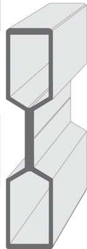
P Z140 Perfil especial 140x30
